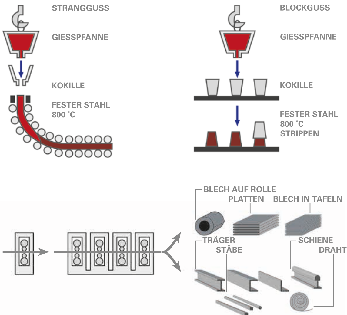
Grafik 7: Vergleich Strangguss- Blockgussverfahren
